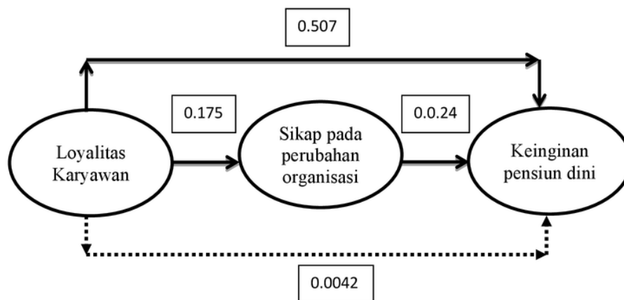
Gambar 2. Uji Mediasi
