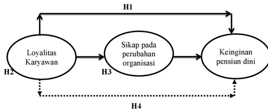
Gambar 1. Kerangka Berpikir
